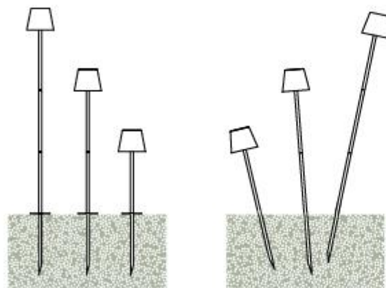
Esempio installazione con disco Example of installation with metal plate
